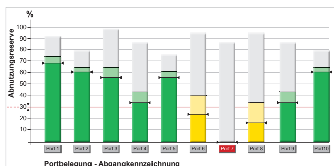
Diagramm zur Online-Leitungsdiagnose
