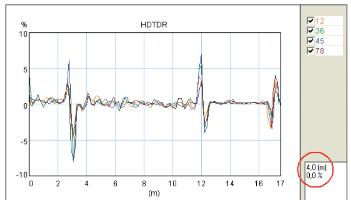
Leitungstester ETHERtest V5.1
