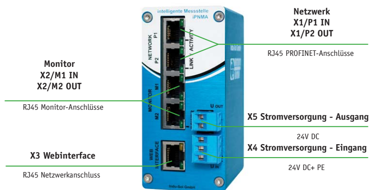
Geräteanschlüsse
