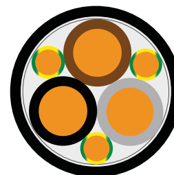
Kabelquerschnitt
